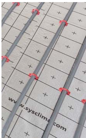
Tubo 16 y grapa 3D.
