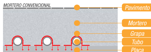
ALU-PS 10, una placa combinable con diferentes tipos de aislamiento.
