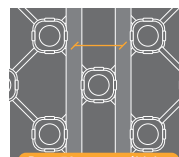
Paso 50 mm y múltiplos
