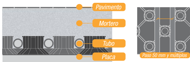
Aislamiento térmico y acústico en modelos NTG.
