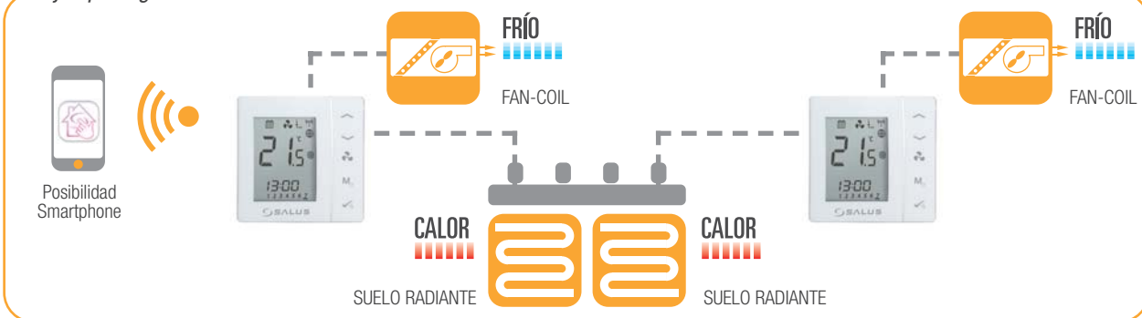
Ejemplo regulación suelo radiante / fan-coil con un solo control
