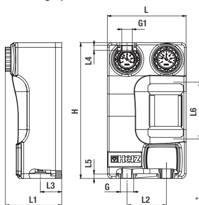
Dimensiones grupos hidráulicos calefacción
