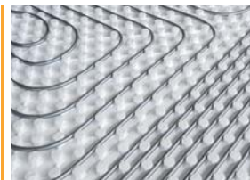
Instalación de tubo con paso a múltiplos de 50 mm.
